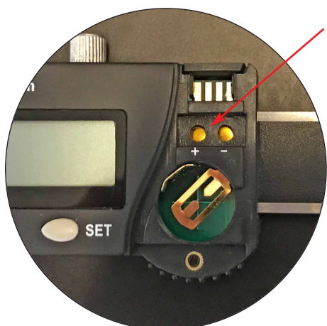
Einstellpunkte Adjust-points
